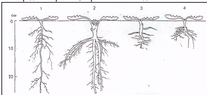
Рисунок 2.1. Изменение направления роста корней у одуванчика ( Taraxacum ) в зависимости от уровня грунтовых вод (по Шуберт, 1988): 1 – сухой луг; 2 – свежий; 3 – сырой луг; 4 – заболоченная территория.
